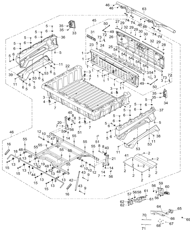
DIAGRAM 2026 CARGO BOX F20-Part 3
