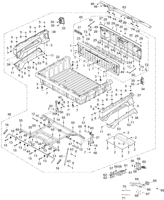
DIAGRAM 2026 CARGO BOX F20-Part 2
